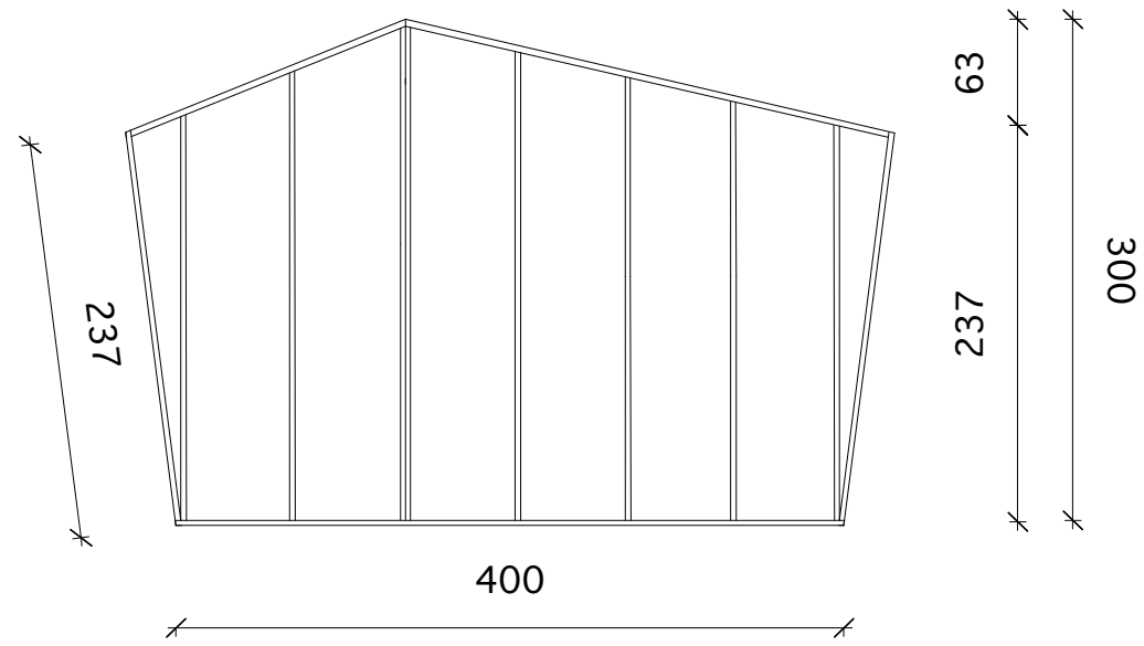
telaio supporto perline
