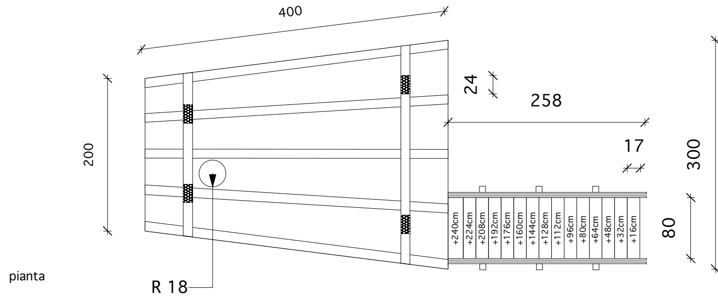
posizionamento struttura portante
